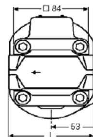
UNA 14h/UNA 16h gniazda gwintowane, UNA 16h gniazda do spawania
