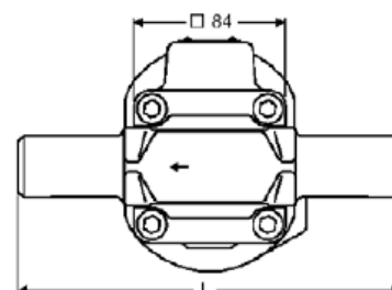
UNA 16h końcówki do spawania
